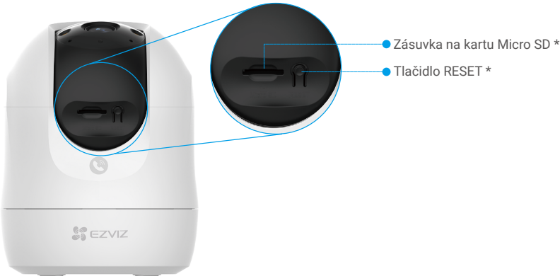
Predné zobrazenie/zadučné zobrazenie
